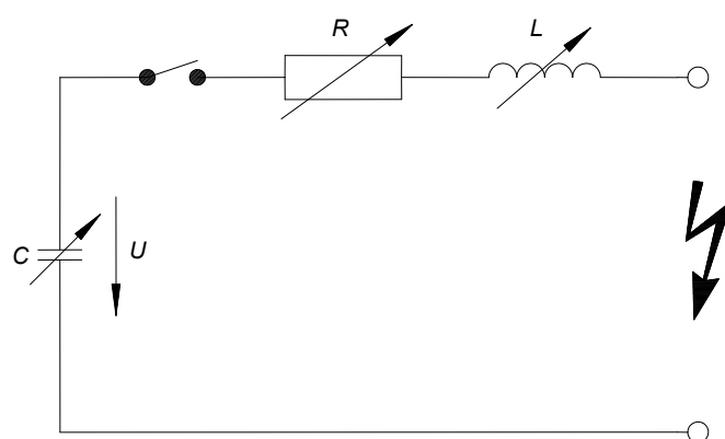
Figure A.13a – Dispositif d'essai
