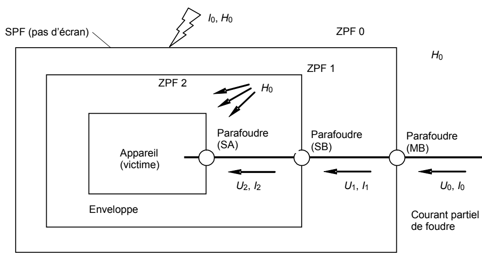
Figure 2d – MPF utilisant seulement une protection coordonnée par parafoudres – Matériels protégés contre les chocs conduits ( U_2 < U_0 et I_2 < I_0 ), mais pas contre les champs magnétiques rayonnés ( H_0 )
