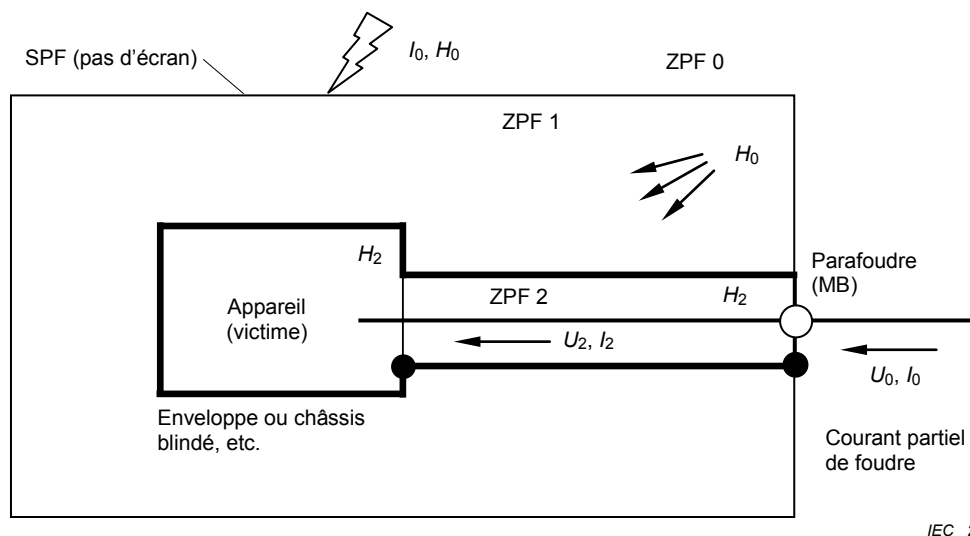
Figure 2c – MPF utilisant un écran de ligne intérieure et une protection par parafoudre à l'entrée de la ZPF 1 – Matériels protégés contre les chocs conduits ( U_2 < U_0 et I_2 < I_0 ) et contre les champs magnétiques rayonnés ( H_2 < H_0 )
