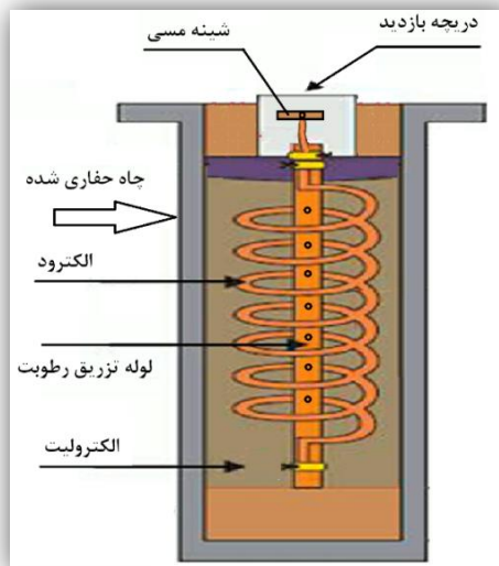
شکل (۶-۲): اجرای الکتروود سیمی به صورت فنی با حداقل ۵ دور سیم مسی با مقطع حداقل ۳۵ میلی‌متر مربع در محیط یک استوانه فرضی به قطر حدود ۵۰ سانتی‌متر
